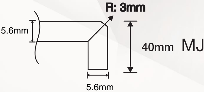
Mitre-Joint
