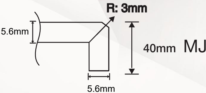
Mitre-Joint
